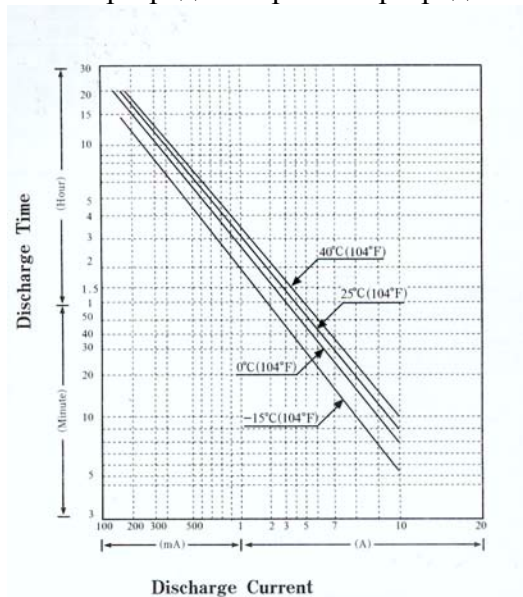
Ток разряда от времени разряда.
